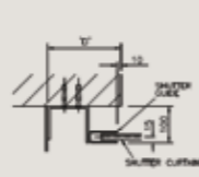
Duvar tipi montaj
